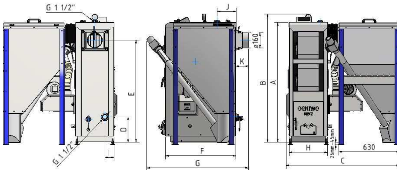
Rys. 4.1 Wymiary kotłów Ogniwo BIO DUO ( z palnikiem, podajnikiem i zbiornikiem paliwa)
