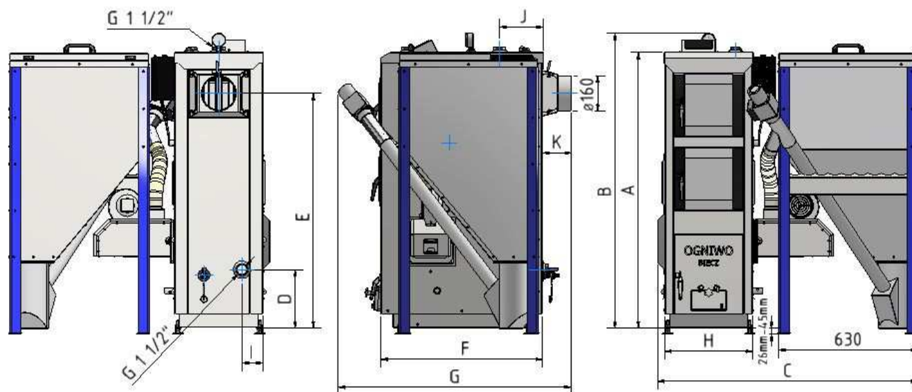
Rys. 4.1 Wymiary kotłów Ogniwko BIO DUO ( z palnikiem, podajnikiem i zbiornikiem paliwa)
