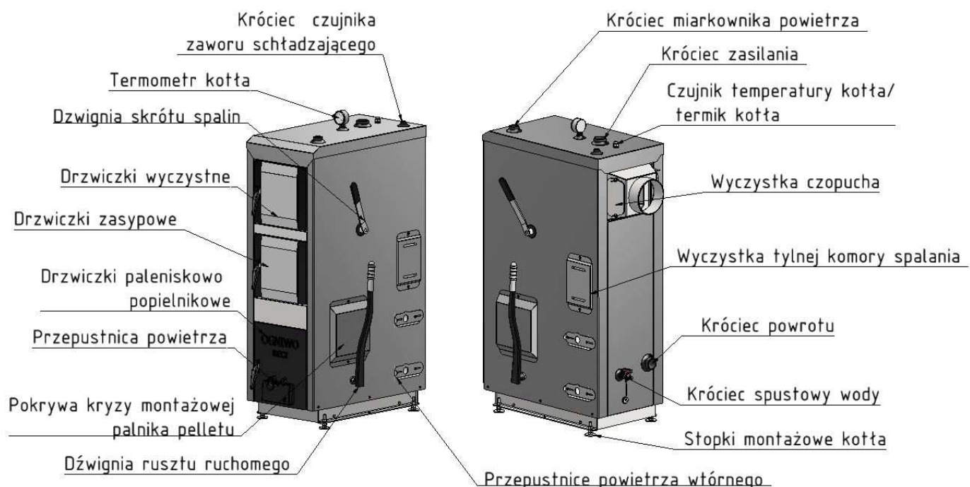
Rys. 3. Podstawowe podzespoły kotła Ogniwio BIO (wersja bez zamontowanego palnika pelletowego)
