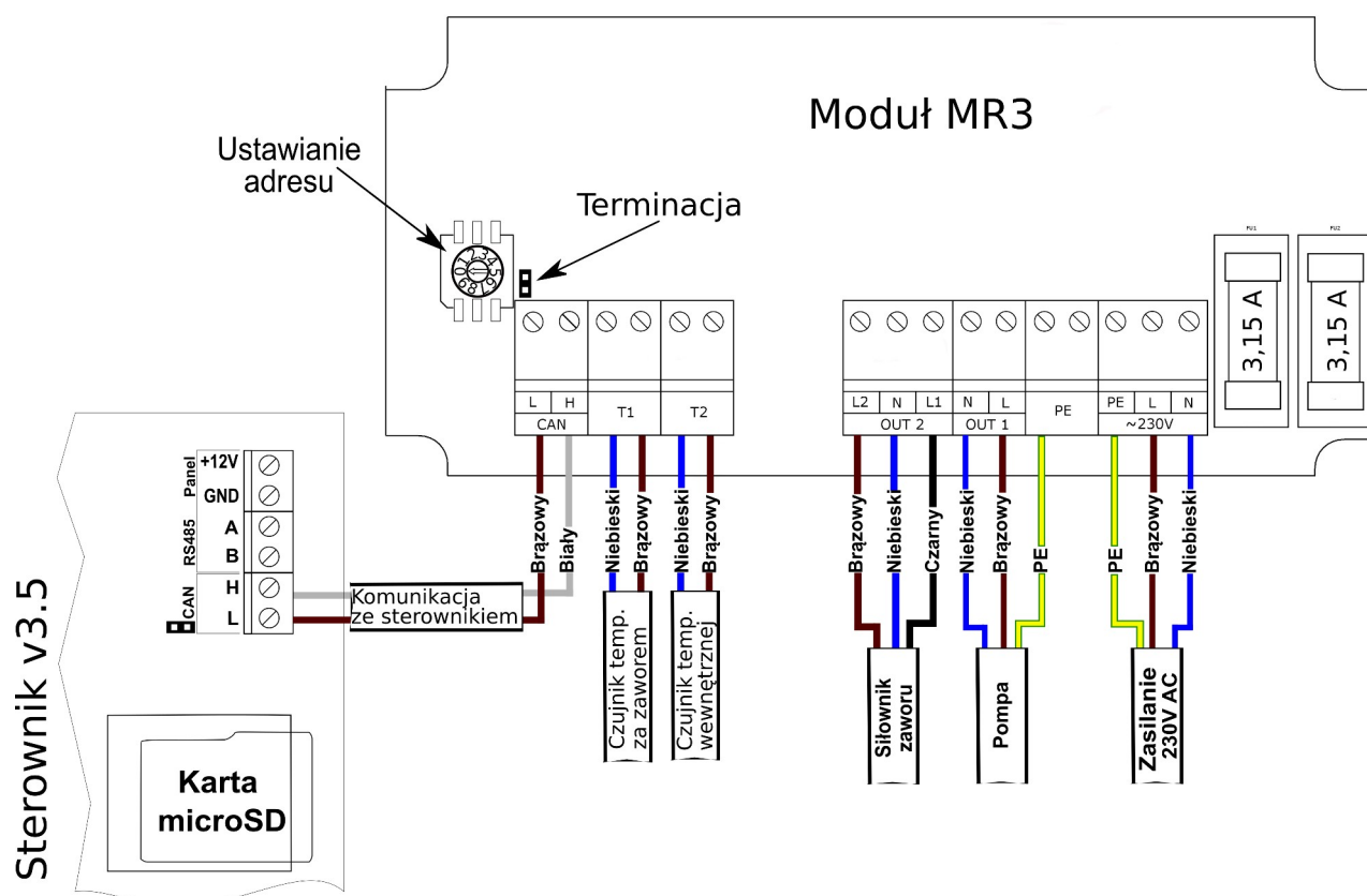
Ilustracja 7: Schemat podłączenia modułu rozszerzeń MR3.
