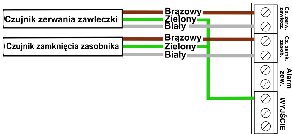
Ilustracja 3: Podłączenie czujników: zerwania zawleczonej oraz zamknięcia zasobnika
