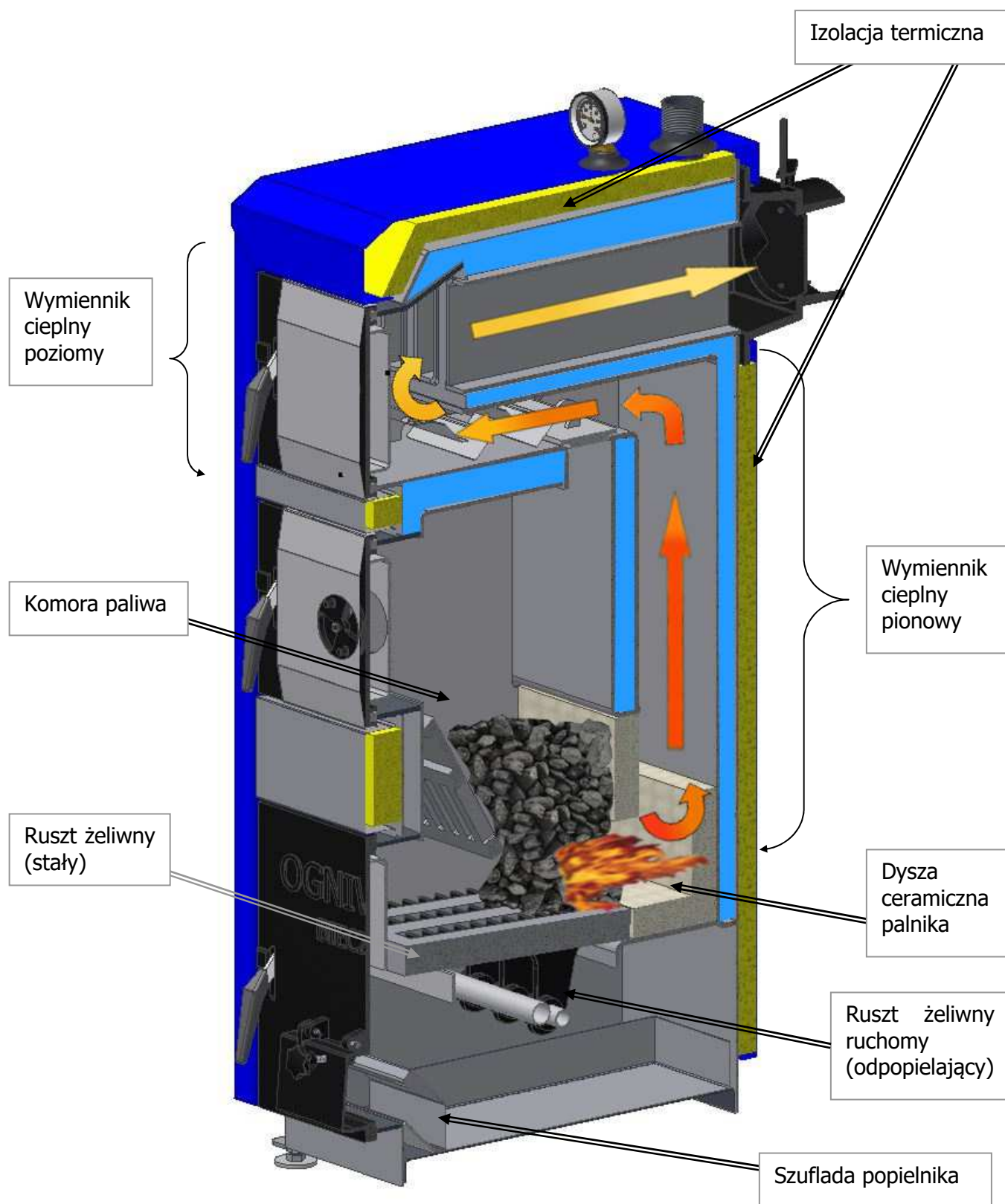
Rys. 1. Obieg spalin w kotle Classic DS
